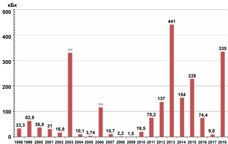
Рис. 2.175. Динамика годовых выбросов ^{137}\text{Cs} в атмосферу в ФГУП «НИТИ им. А. П. Александрова» за 1998-2018 годы
