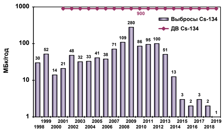
Рис. 2.125. Динамика годовых выбросов ^{134}\text{Cs} в атмосферу, НВАЭС
