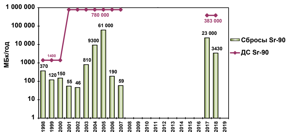
Рис. 2.133. Динамика годовых сбросов радионуклидов ^{90}\text{Sr} со сточными водами в бассейн Дона (за 2017 и 2018 годы даны сбросы только с НВАЭС-2)
