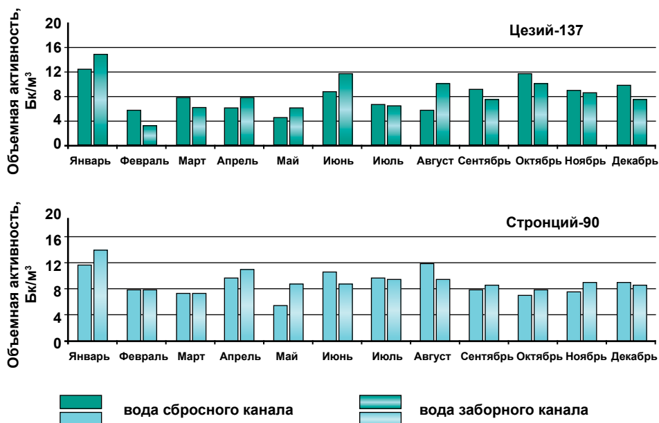
Рис. 2.177. Содержание техногенных радионуклидов в заборной и сбросной воде ФГУП «НИТИ им. А. П. Александра» в течение 2012 года [12]
