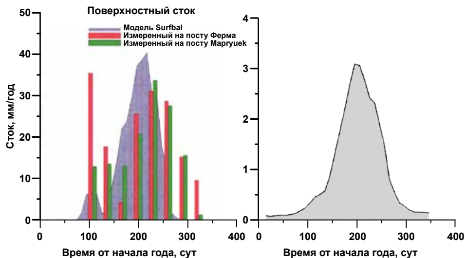
Рис. 2.9. Модельный среднемноголетний гидрограф стока за 1947-2012 годы при номере кривой стока 72 (годовая сумма — 9 мм) и среднемесечный сток реки Урулюнгуй, измеренный на гидропостах (рисунок слева); среднемноголетнее внутригодовое распределение интенсивности осадков (рисунок справа) [7]
