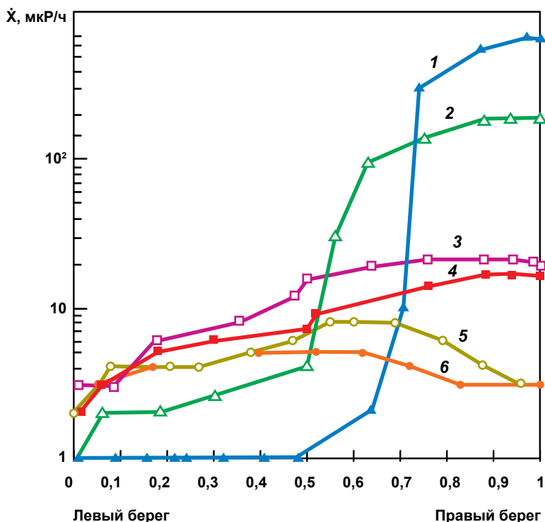
Рис. 2.82. Распределение мощности дозы \gamma -излучения воды в поперечном сечении Енисея на расстояниях 0,15 (1), 3 (2), 16 (3), 25 (4), 57 (5), 104 км (6) от места сброса [52]
