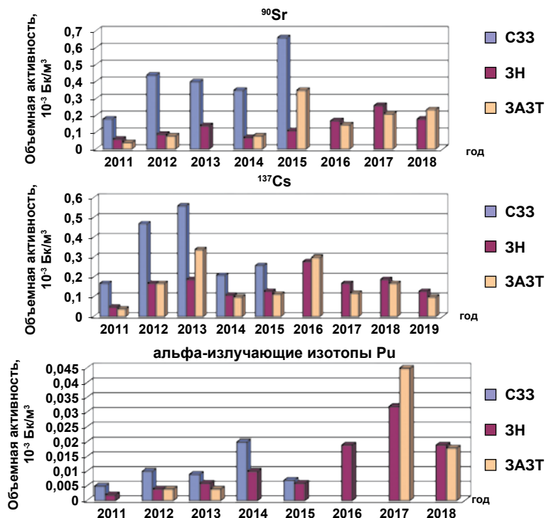
Рис. 2.55. Динамика изменений объемной активности ^{90}\text{Sr} , ^{137}\text{Cs} и Pu в приземном воздухе в регионе ПО «Маяк»
