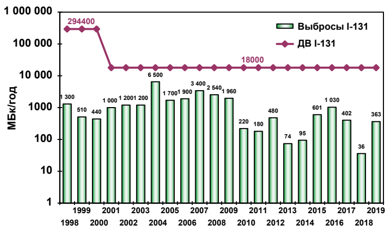
Рис. 2.126. Динамика годовых выбросов ^{131}\text{I} в атмосферу, НВАЭС
