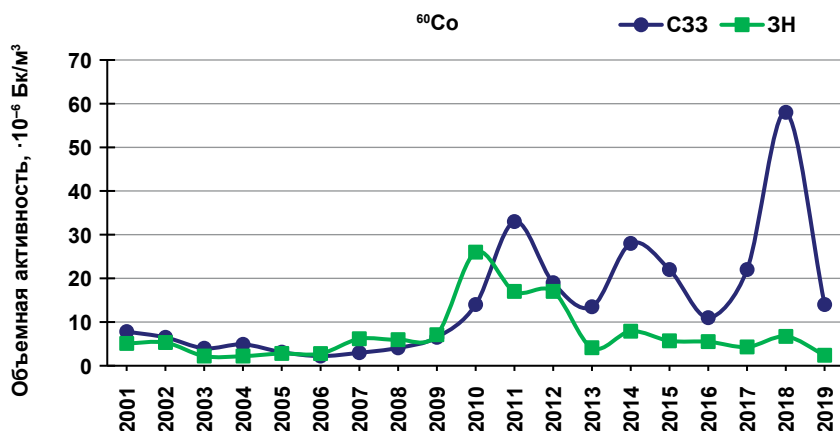
Рис. 2.186. Среднегодовая объемная активность ^{60}\text{Co} в приземном слое атмосферы СЗЗ и ЗН ЛАЭС в 2001-2019 годах
