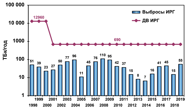
Рис. 2.124. Динамика годовых выбросов ИРГ в атмосферу, НВАЭС
