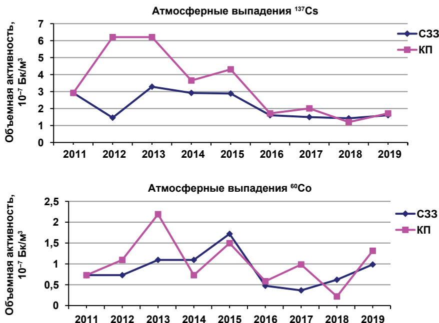
Рис. 2.139. Динамика плотности атмосферных выпадений ^{60}\text{Co} и ^{137}\text{Cs} в С33 и КП НВАЭС
