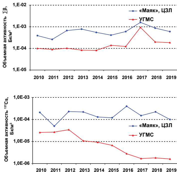
Рис. 2.57. Динамика объемной активности \Sigma\beta и ^{137}\text{Cs} в приземном слое атмосферы п. Новогорный по данным ЦЗЛ ПО «Маяк» и Уральского УГМС
