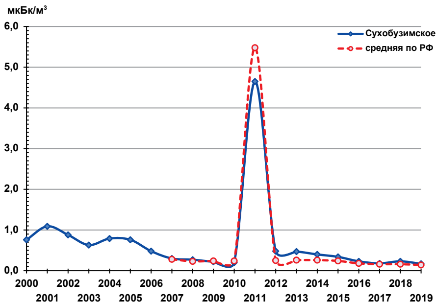
Рис. 2.87. Средняя за год концентрация ^{137}\text{Cs} в воздухе, измеренная на посту в п. Сухобузимское и в РФ
