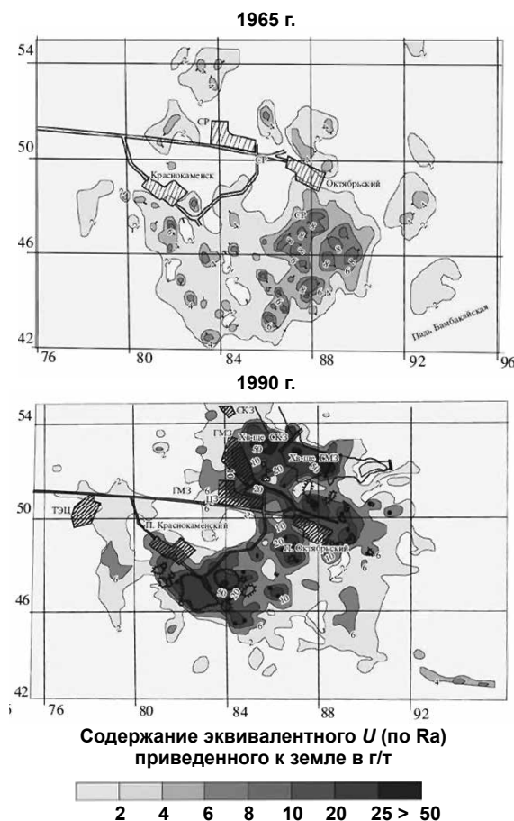
Рис. 2.24. Содержание эквивалентного урана в почвах Стрельцовского рудного поля в 1965 и 1990 годах (по материалам ППГХО)
