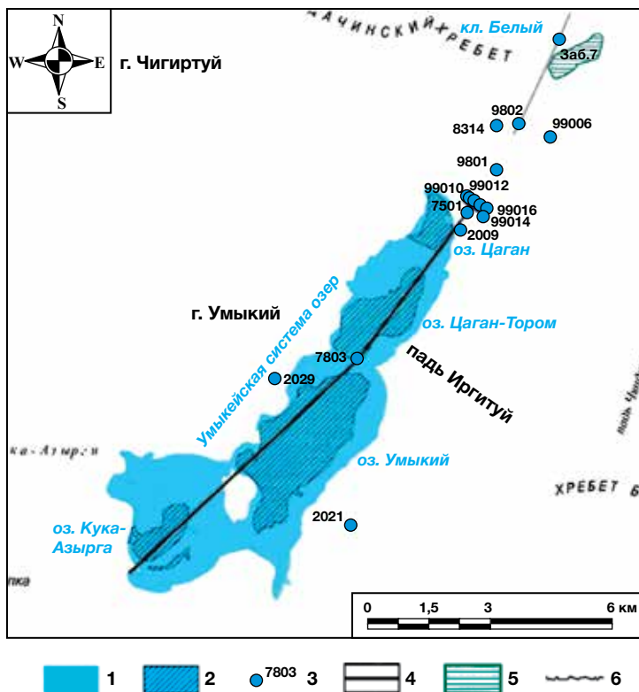
Рис. 2.13. Схема современного состояния Умыкейской системы озер [7]: 1 — водоемы; 2 — контуры озер в естественных границах (до затопления); 3 — наблюдательные скважины; 4 — линия профиля через озера; 5 — заболоченности; 6 — гидросооружения: плотины
