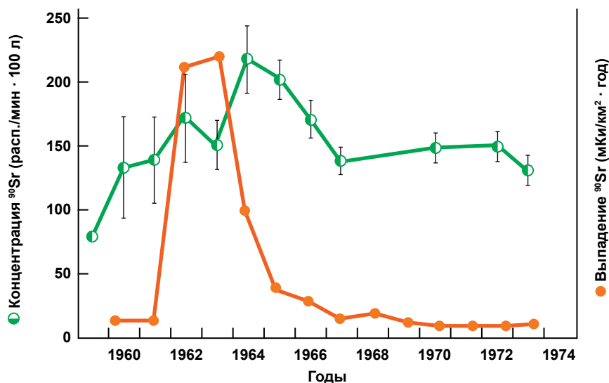
Рис. 2.180. Динамика ^{90}\text{Sr} в водах Балтийского моря и выпадения ^{90}\text{Sr} на поверхность с 1959 по 1973 годы (рисунок из доклада [111], единицы измерения сохранены, как в оригинале: 180 расп./мин на 100 л равны 30 Бк/м³)
