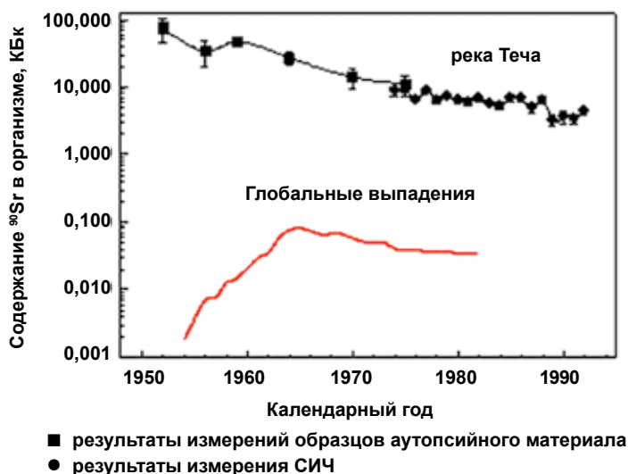
Рис. 2.71. Динамика содержания ^{90}\text{Sr} в организме взрослых жителей с. Муслюмово в сравнении с глобальными уровнями [161]
