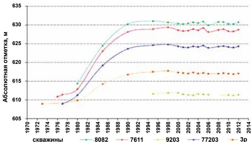
Рис. 2.19. Динамика уровней подземных вод в падах Широңдукуй и Сухой Урулунгуй за период с 1973 по 2012 годы [7]
