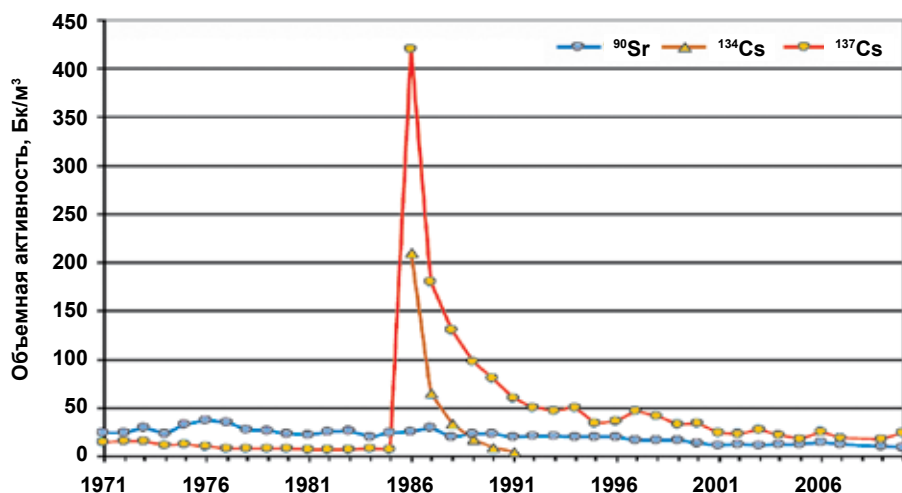
Рис. 2.179. Динамика концентраций радионуклидов в Копорской губе с момента начала исследований [105]
